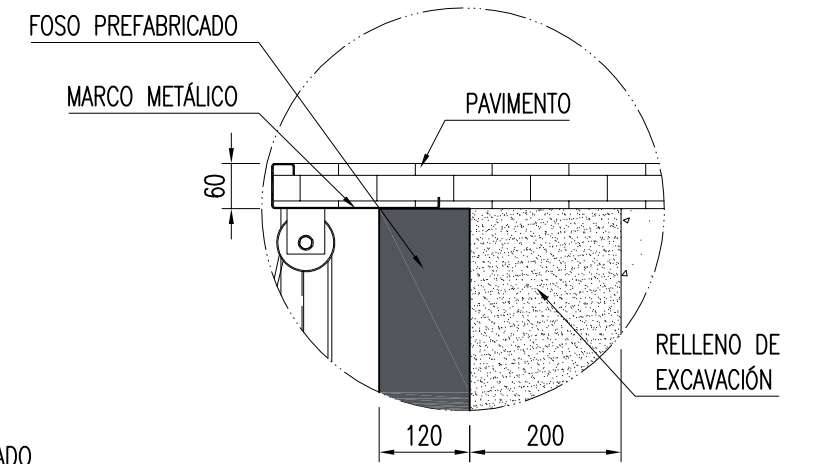
DETALLE "B"
